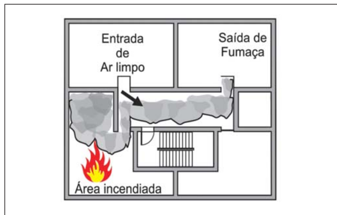
Figura 20: Extração mecânica
