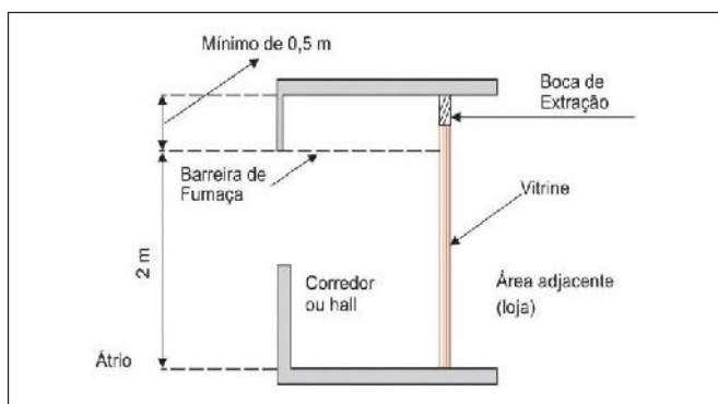
Figura 7: Detalhe de barreira de fumaça – corte
