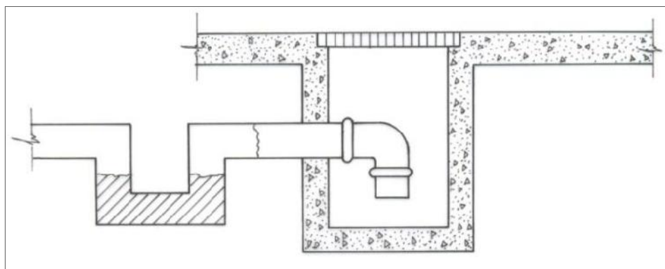
Figura 4.24: Detalhes de purgador selado por líquido.
