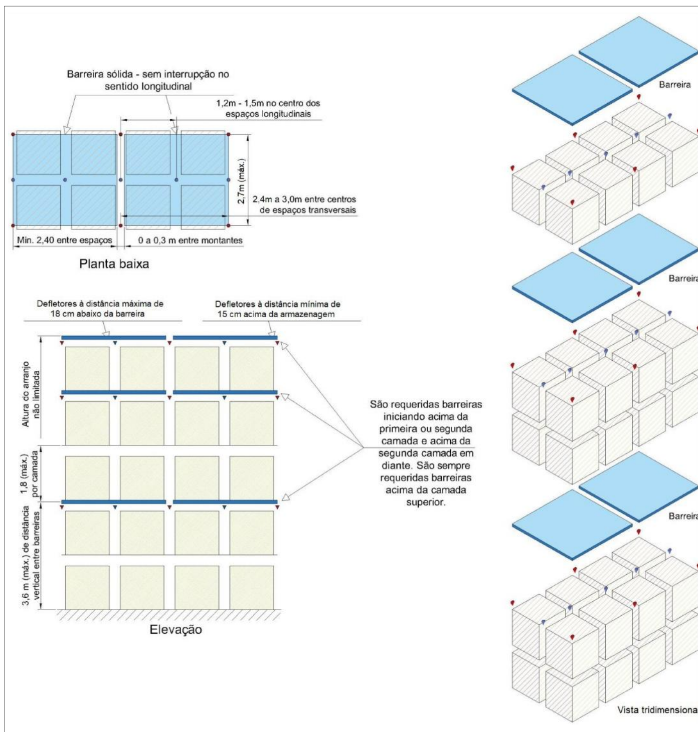
Figura 4.13: Leiaute de chuviros automáticos para estrutura-suporte de fileira dupla – Esquema de projeto "C".
