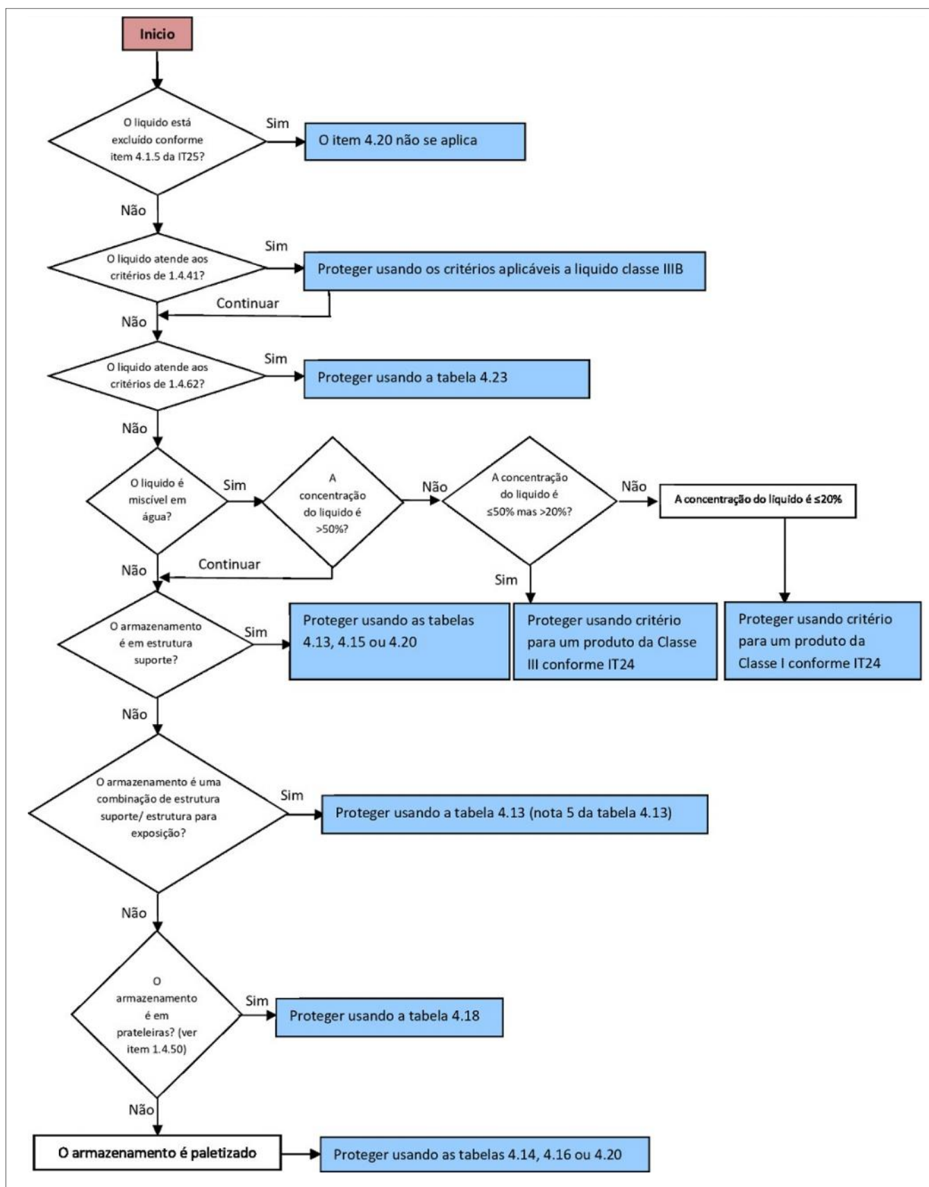
Figura 4.2: Árvore de decisão para o critério de proteção para recipientes metálicos contendo líquidos miscíveis e não miscíveis em água – Inflamável e combustível.
