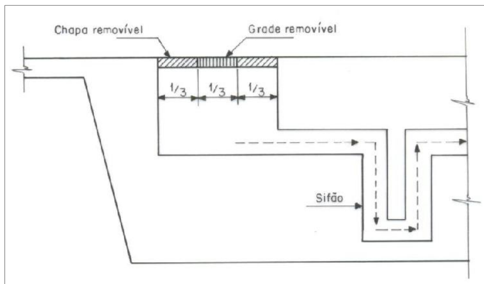
Figura 4.22: Detalhes do projeto de drenagem de canalatas.
