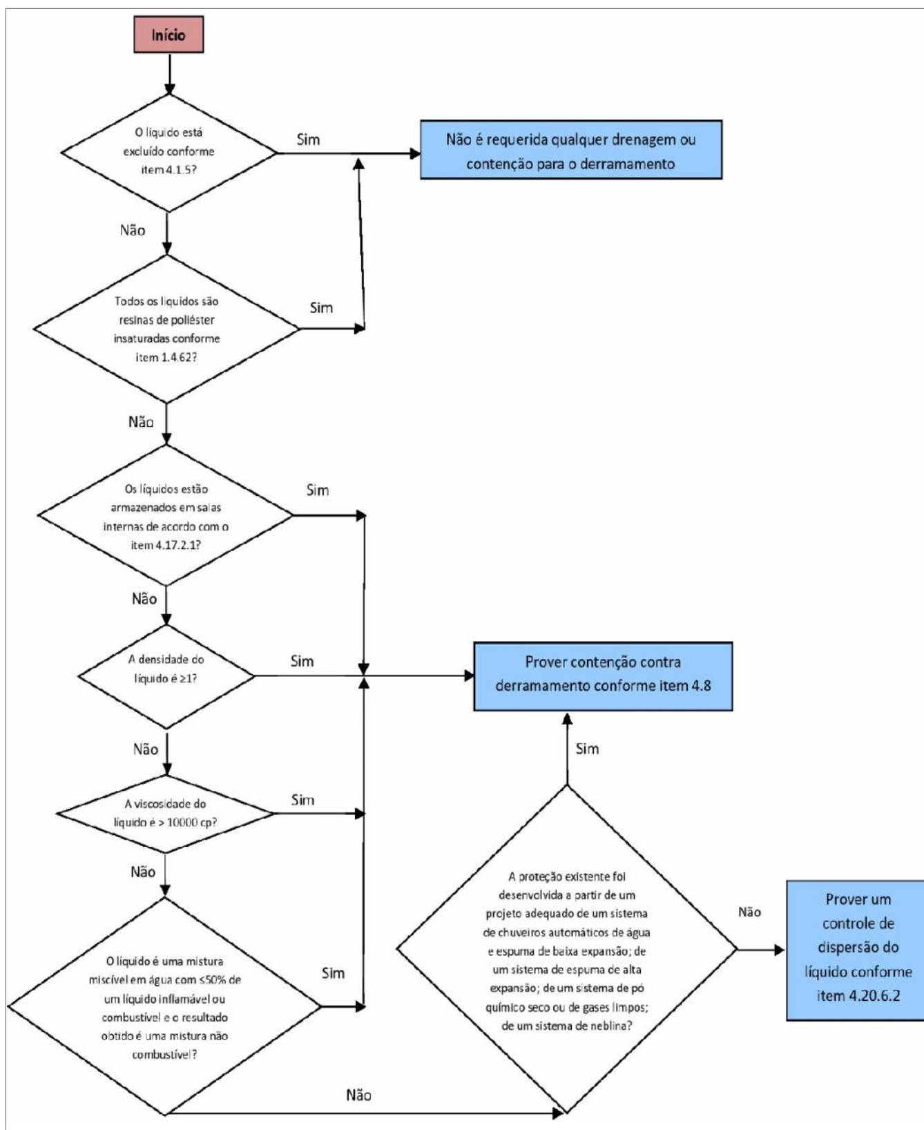
Figura 4.5: Contenção de derramamentos e controle de dispersão de líquidos em áreas de armazenamento protegidas.
