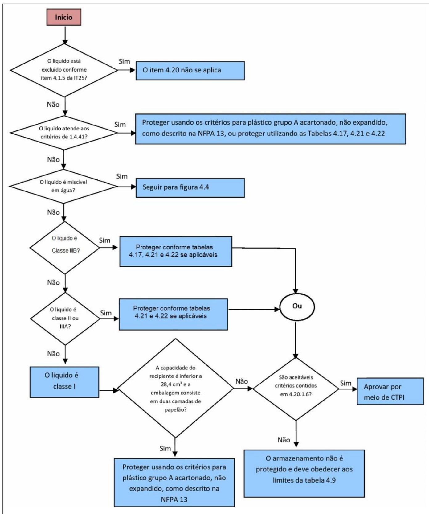
Figura 4.3: Árvore de decisão para o critério de proteção para recipiente não metálico contendo líquidos miscíveis e não miscíveis em água – Inflamável e combustível.
