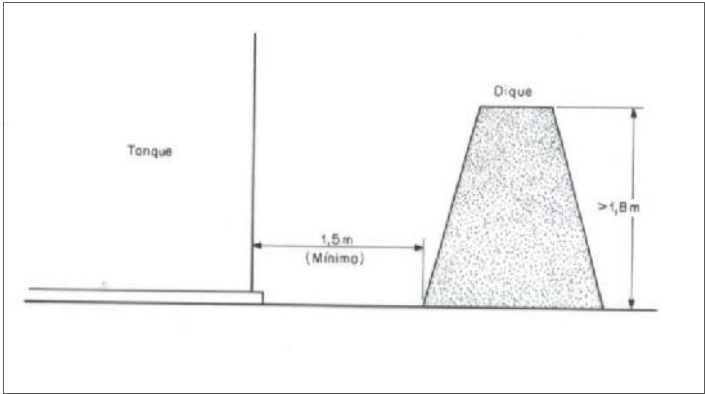
Figura 2.2: Distância mínima entre o costado do tanque e a face do dique
