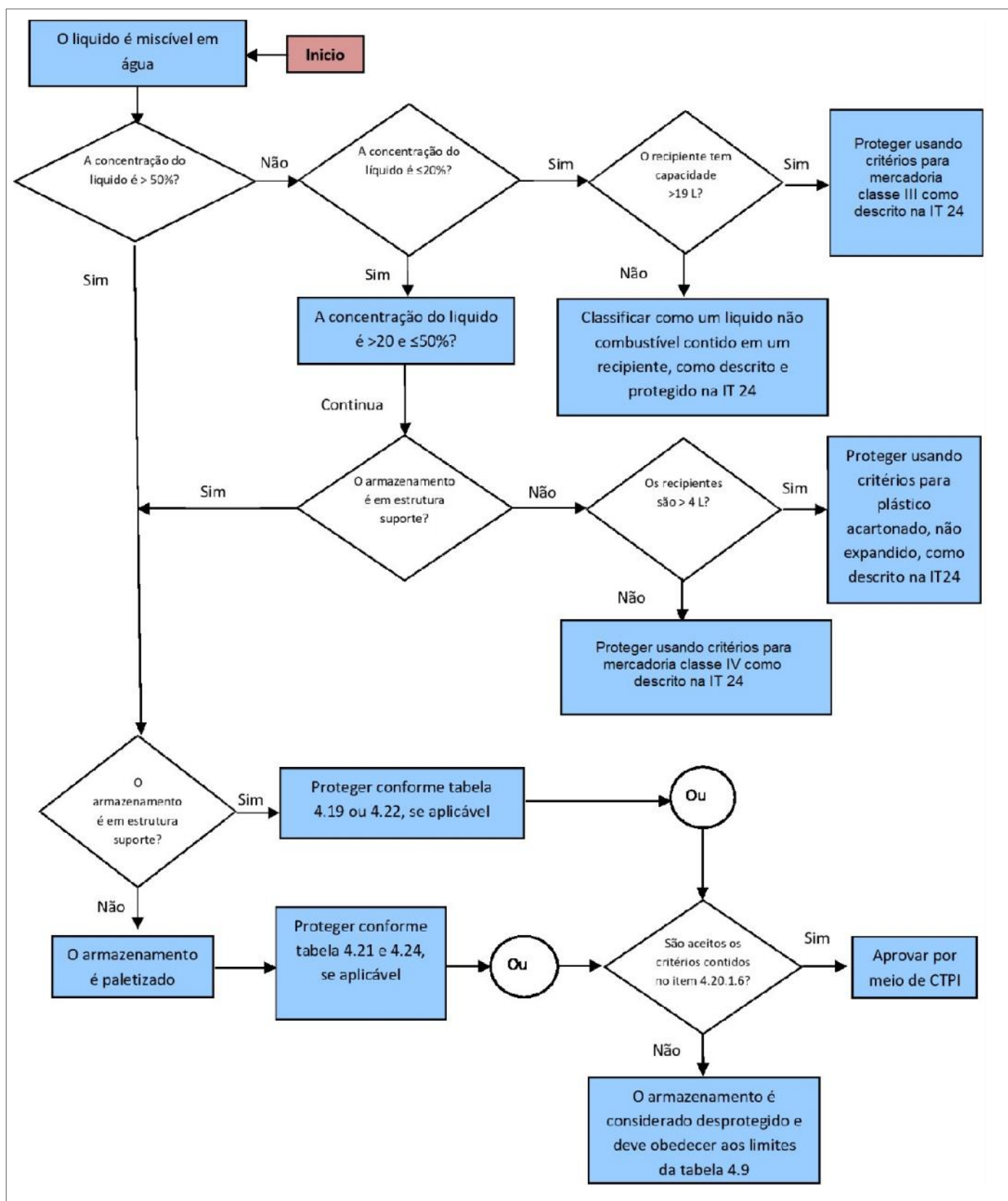
Figura 4.4: Árvore de decisão para o critério de proteção contra incêndio para líquidos inflamáveis e combustíveis miscíveis em água contidos em recipientes não metálicos.
