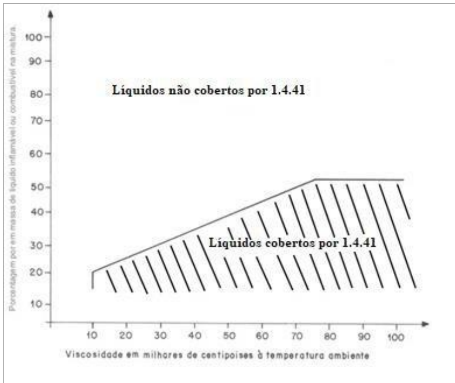
Figura 4.1: Viscosidade versus concentração porcentual em massa de componente inflamável ou combustível.
